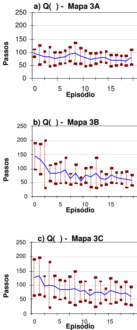
Figura 16: Curvas de aprendizagem para Q(\lambda) , mapa 3. Particionamento: a) Original b) Perfeito c) Pior.
