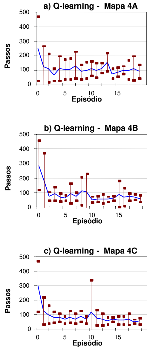
Figura 17: Curvas de aprendizagem para Q-learning, mapa 4. Particionamento: a) Original b) Perfeito c) Pior.
