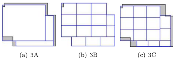
Figura 7: Mapa 3: sala com dois obstáculos nos cantos. Versões de particionamento: a) 3A (Original), b) 3B (Perfeito), c) 3C (Pior).
