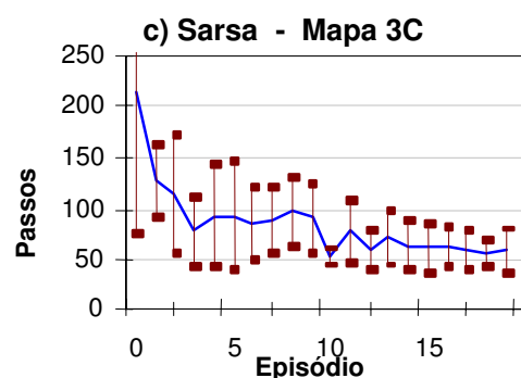
Figura 15: Curvas de aprendizagem para Sarsa, mapa 3. Particionamento: a) Original b) Perfeito c) Pior.
